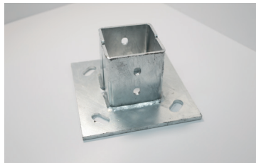
BASE FRAME(용융아연도금(HDG)) 구조물 수직 기둥(Post) 하부 지지 및 콘크리트 기초 양카 고정부
